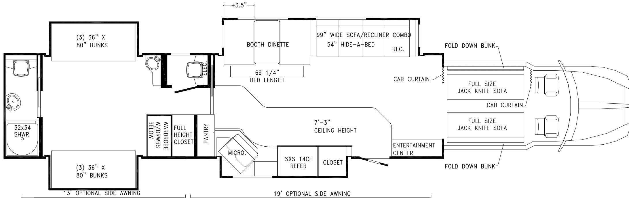
2006 - 52' 4 SLIDE-OUT 770/780 (ENTERTAINER UNIT)
